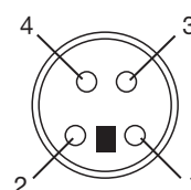
MINI DIN 4-pin
